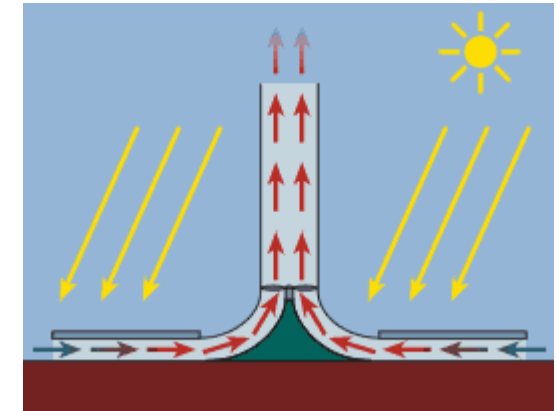
Chimenea solar
